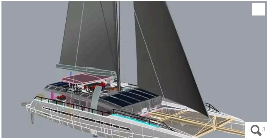
Le bâtiment accueillera la construction d'un catamaran de course-croisière de 125 pieds (38 mètres de long) et de 15 mètres de large pour un poids 80 tonnes, dont 37 de composite carbone. © FC Cube
